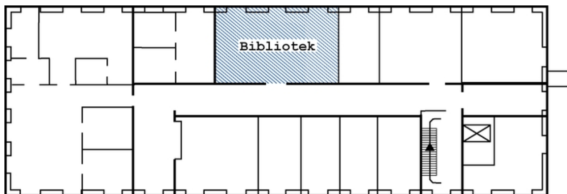
Plantegning 3. etasje.
