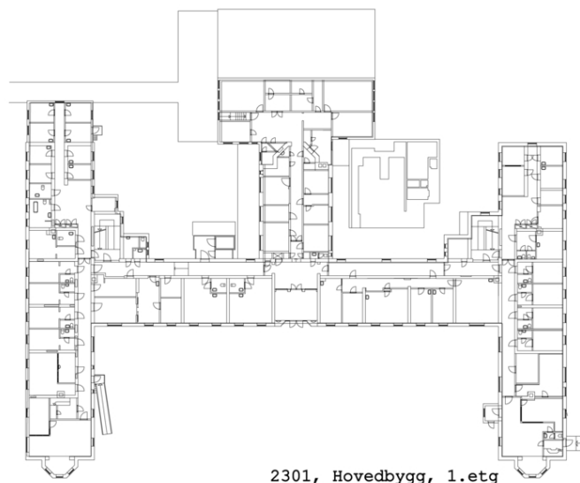
Plantegning 1. etasje.
