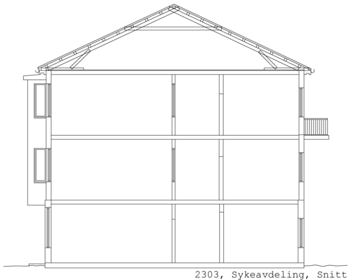
Snitt av bygg 3.
