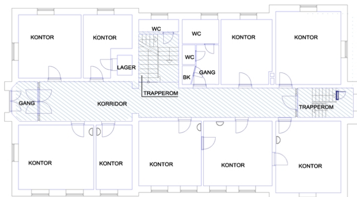
Plantegning 1. etasje.
