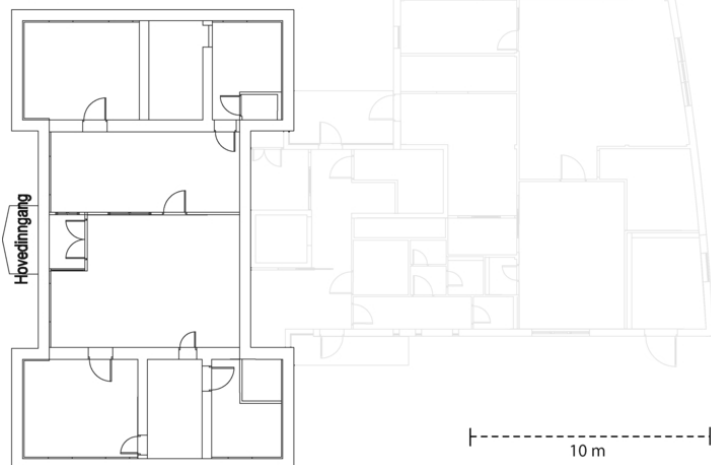
Plantegning 1. etasje.
