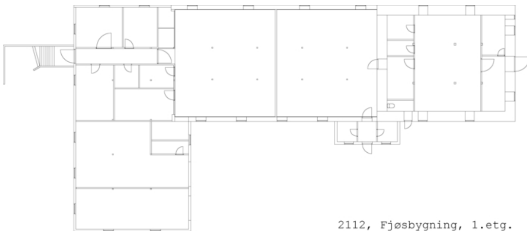
Plantegning bygning 12.
