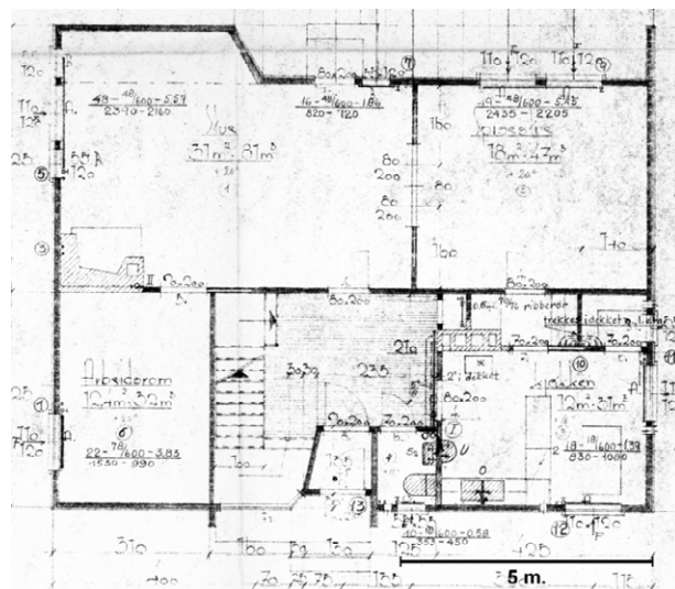
Plantegning 1. etasje.
