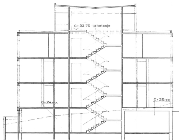
Snittegning av bygningen.
