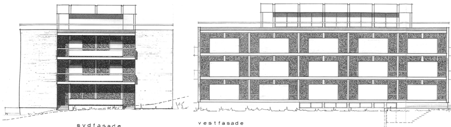
Tegning av sydfasaden.
