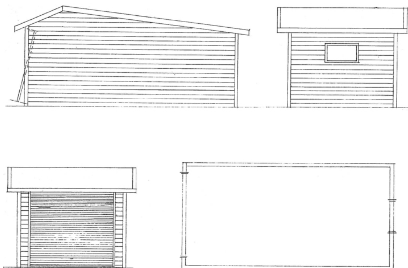
Tegning garasjer for legeboligene.
