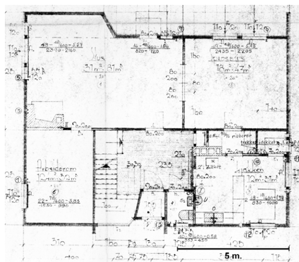
Plantegning 1. etasje.
