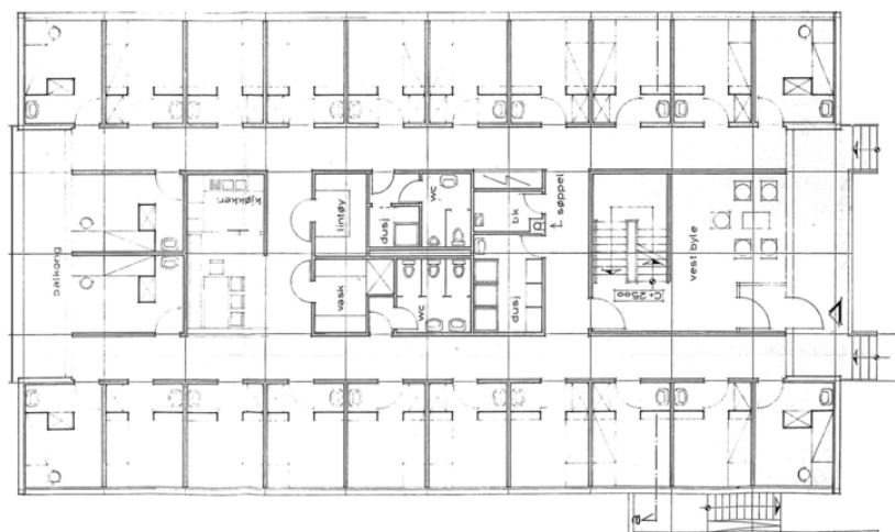
Plantegning 1. etasje.
