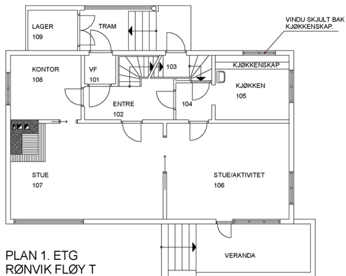
Plantegning 1. etasje.
