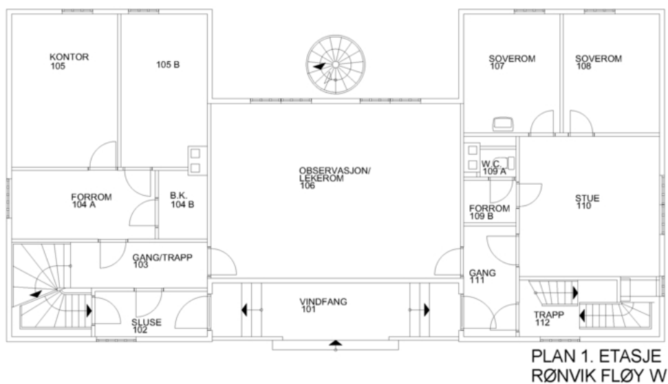
Plantegning 1. etasje.
