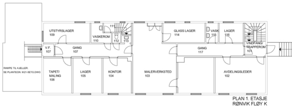
Plantegning 1. etasje.
