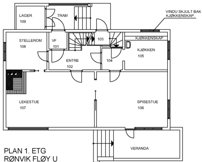
Plantegegning 1. etasje.
