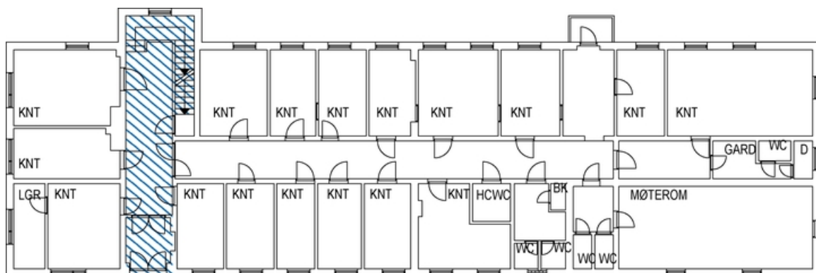
Plantegning 1. etasje.
