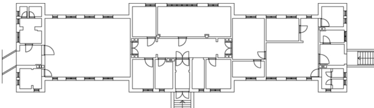
Plantegning 1. etasje.
