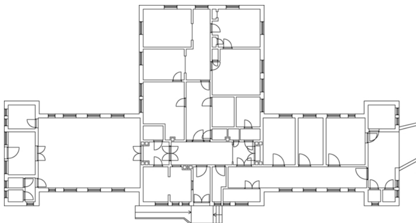
Plantegning 1. etasje.
