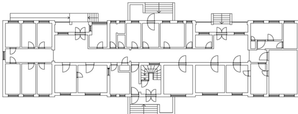
Plantegning 1. etasje.
