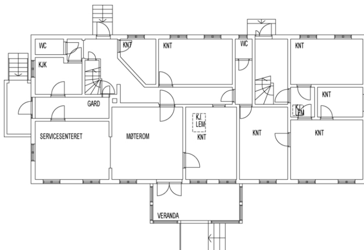
Plantegning 1. etasje.
