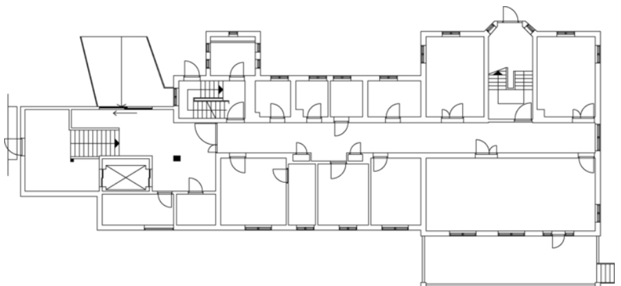
Plantegning 1. etasje.
