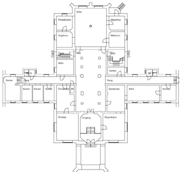
Plantegning 1. etasje.
