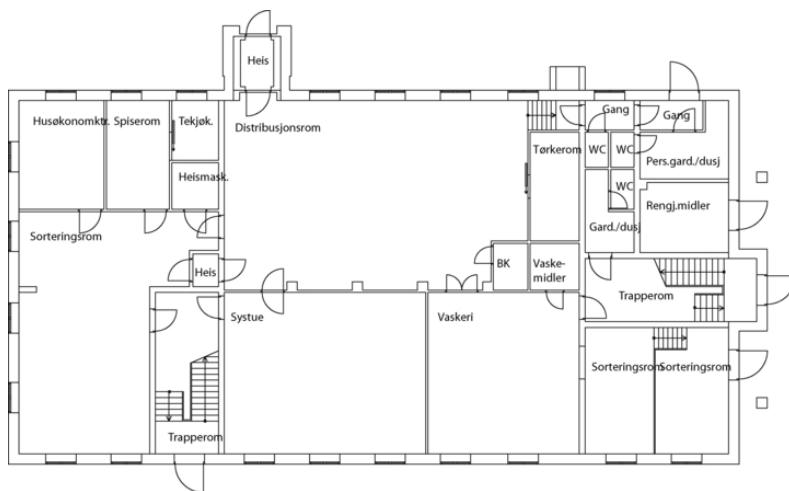
Plantegning 1. etasje.
