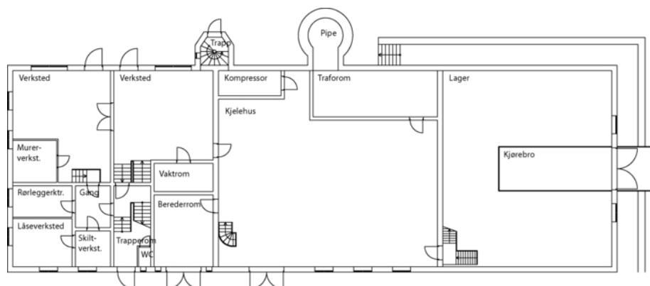
Plantegning 1. etasje.
