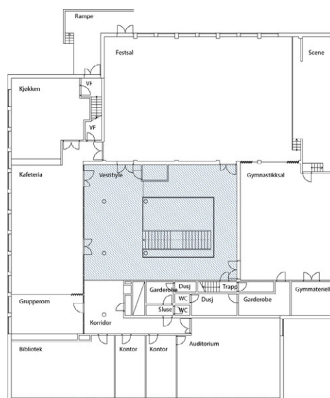
Plantegning 2. etasje.
