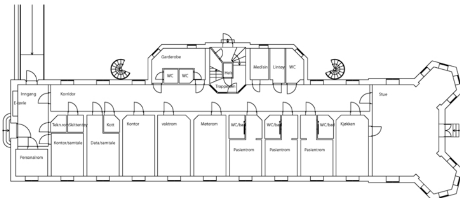
Plantegning 1. etasje.
