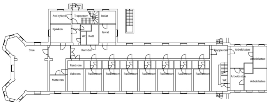
Plantegning 1. etasje.
