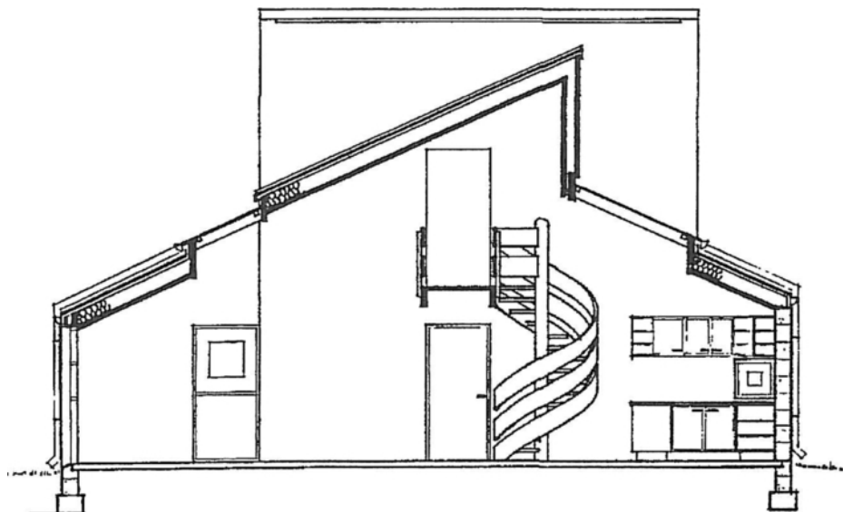
Snittegning av huset.
