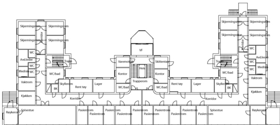
Plantegning 1. etasje.
