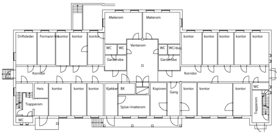
Plantegning 1. etasje.
