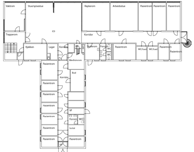
Plantegning 1. etasje.
