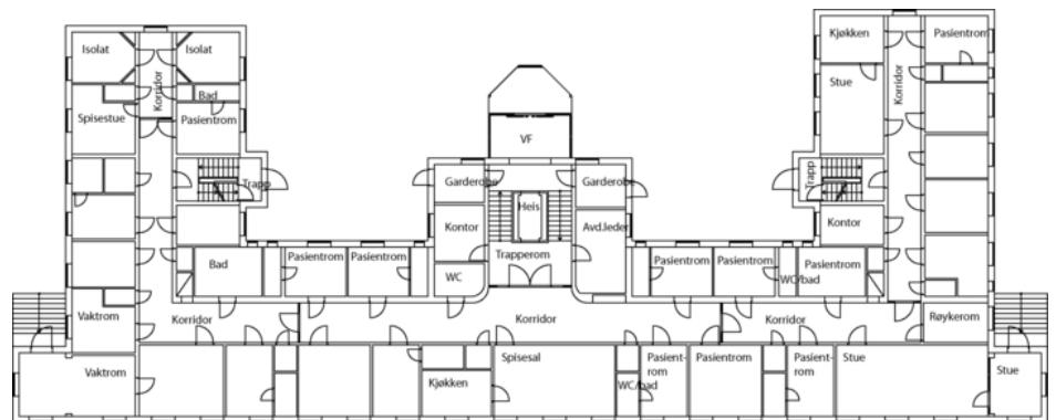
Plantegning 1. etasje.
