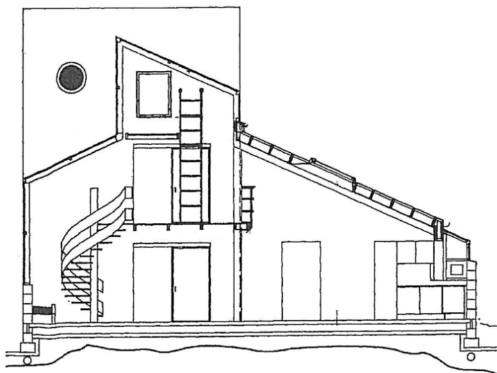
Snittegning.
