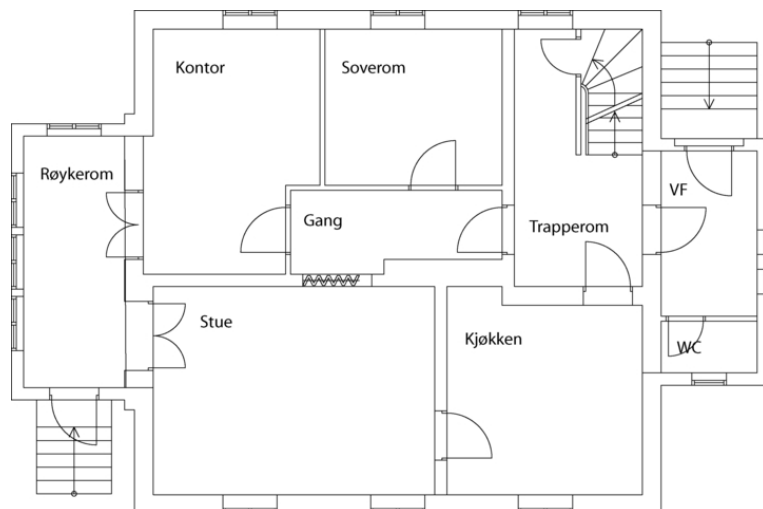
Plantegning 1. etasje.
