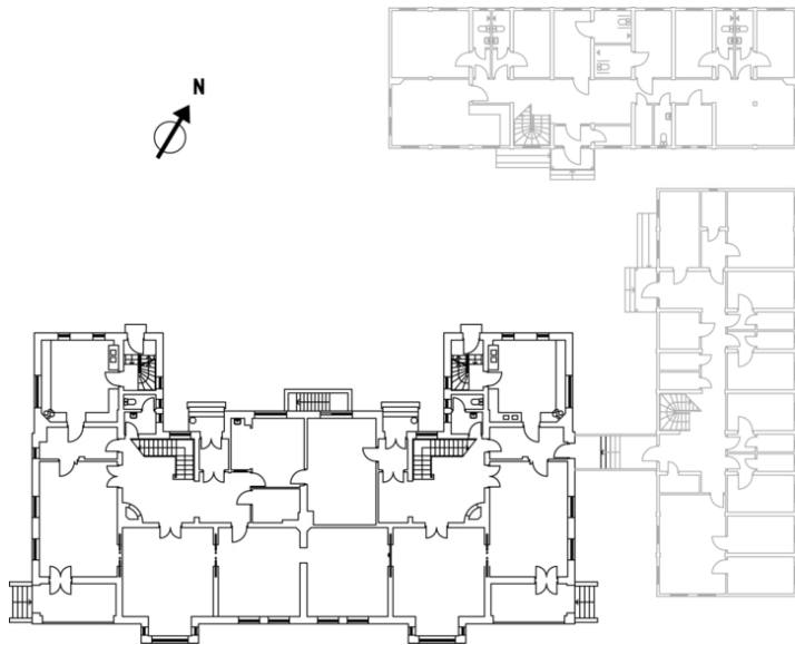
Plantegning 1. etasje.
