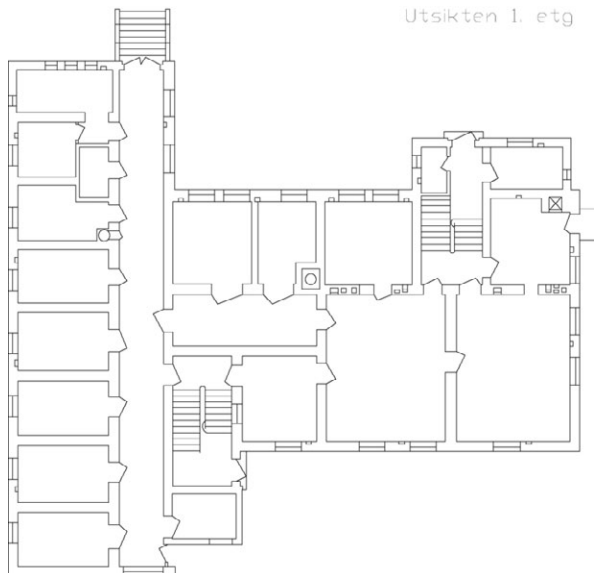
Plantegning 1. etasje.
