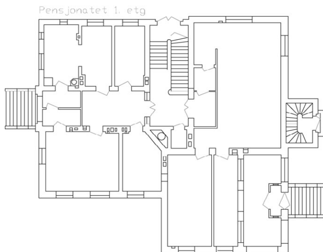
Plantegning 1. etasje.
