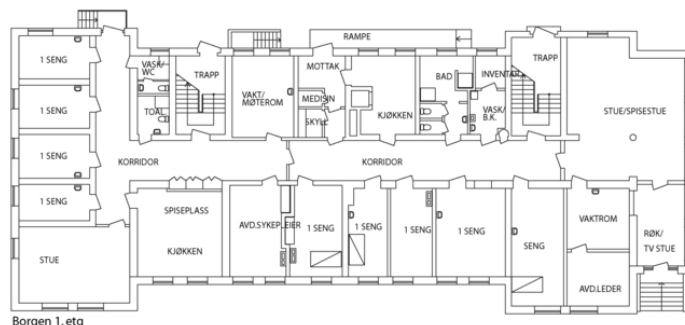
Plantegning 1. etasje.
