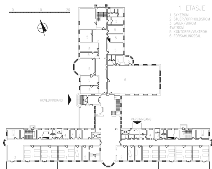
Plantegning 1. etasje.
