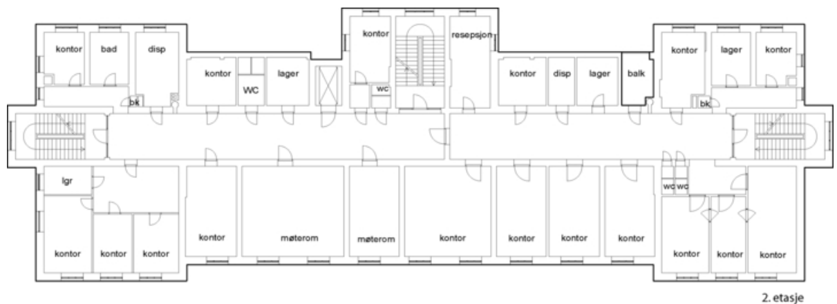
Plantegning 2. etasje.
