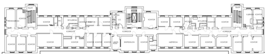
Plantegning 2. etasje.
