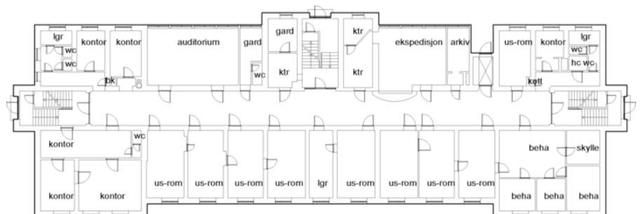
Plantegning 1. etasje.
