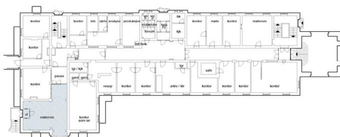
Plantegning 1. etasje.
