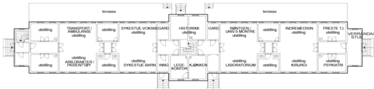
Plantegning 1. etasje.
