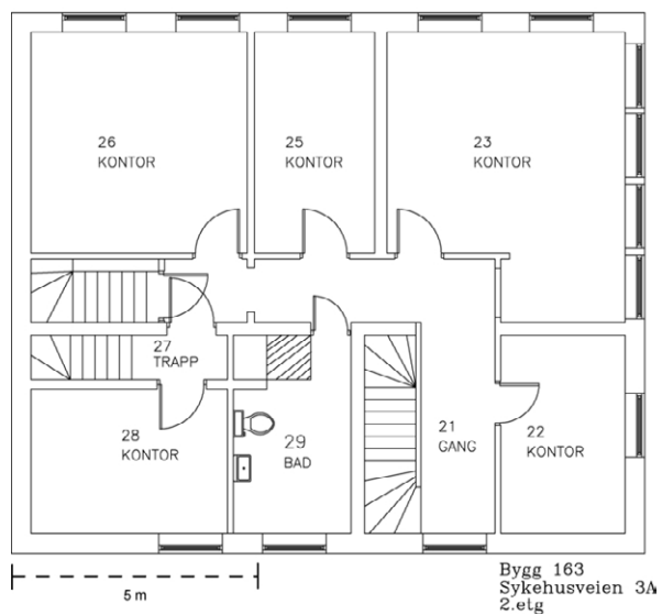
Plantegning 2. etasje.
