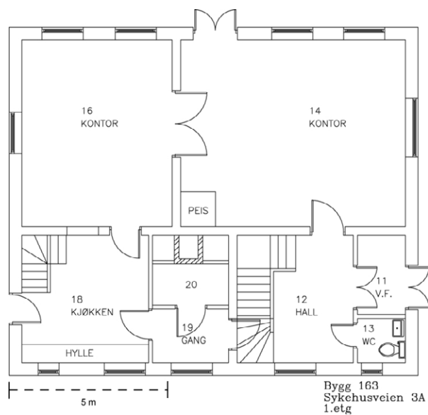
Plantegning 1. etasje.
