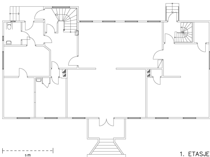
Plantegning 1. etasje.
