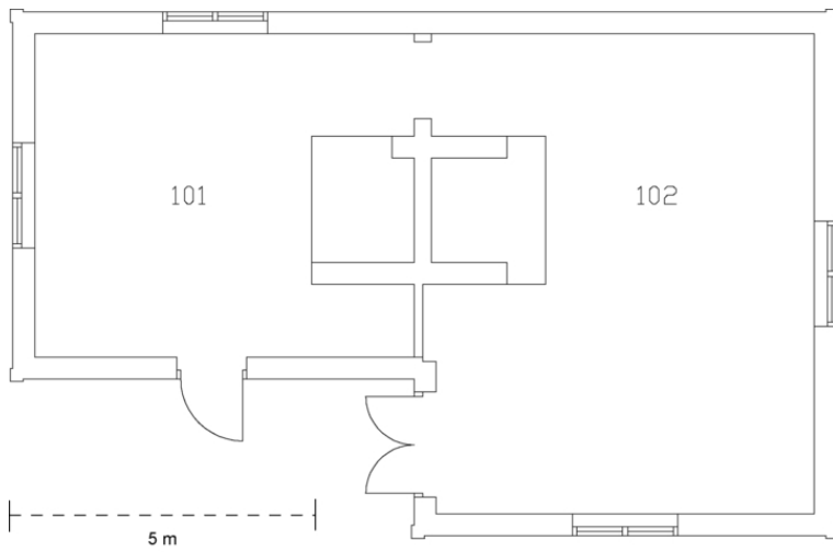
Plantegning bakstehuset.
