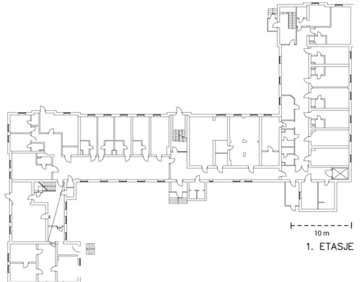
Plantegning 1. etasje.
