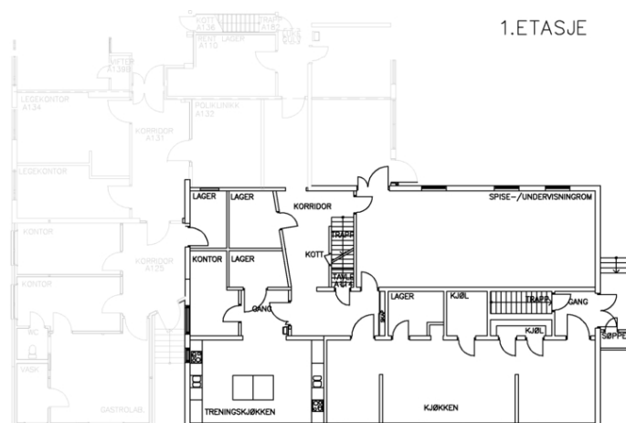
Plantegning 1. etasje.
