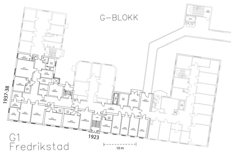
Plantegning 1. etasje, G-blokk I og II.
