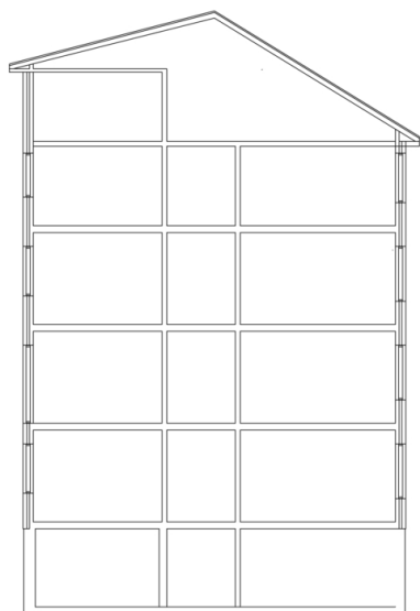
Snittegning, G-blokk II, sett mot nord.
