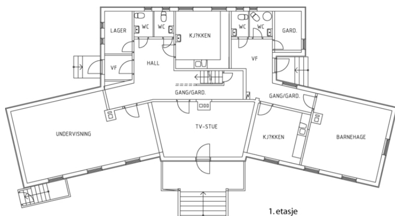
Plantegning 1. etasje.
