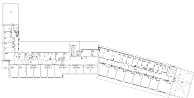
Plantegning 2. etasje.
