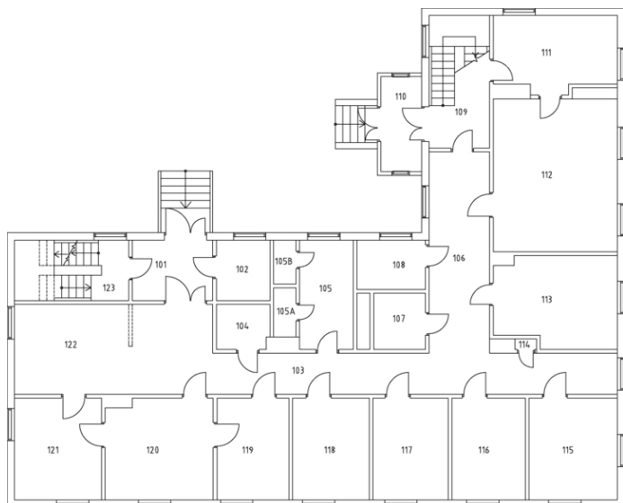
Plantegning 1. etasje.
