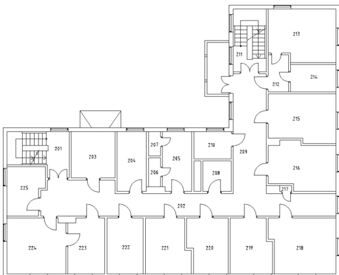
Plantegning 2. etasje.
