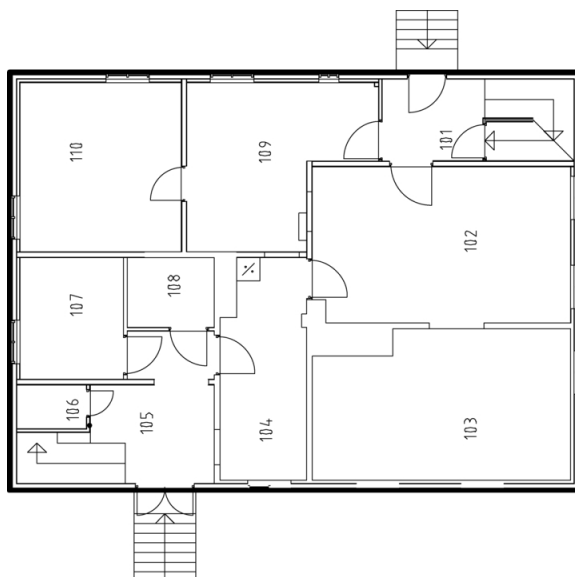
Plantegning 1. etasje.
