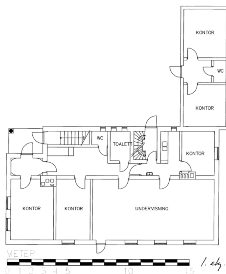
Plantegning 1. etasje.
