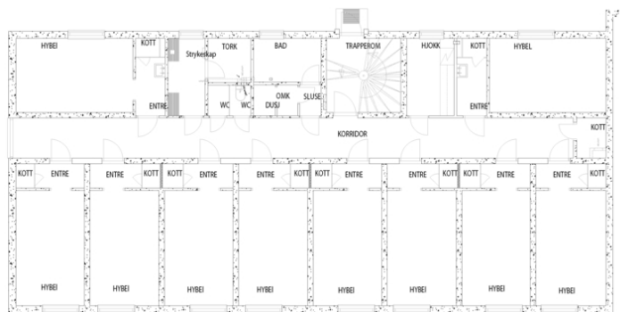
Plantegning 1. etasje, nord.
