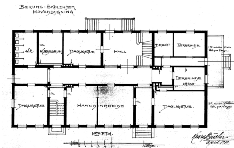
Plantegning 1919, 1. etasje.
