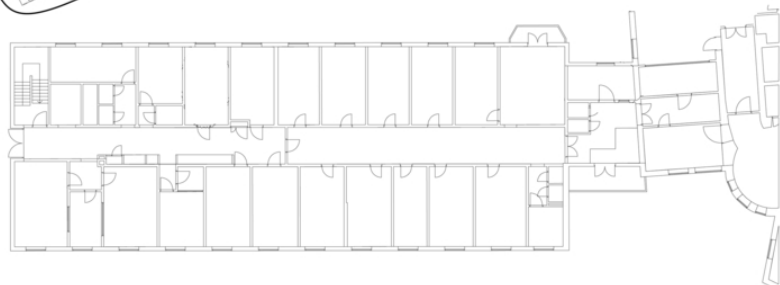
SYDFLØY 1. etasje
