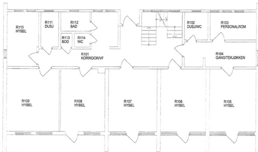
Plantegning 1. etasje.
