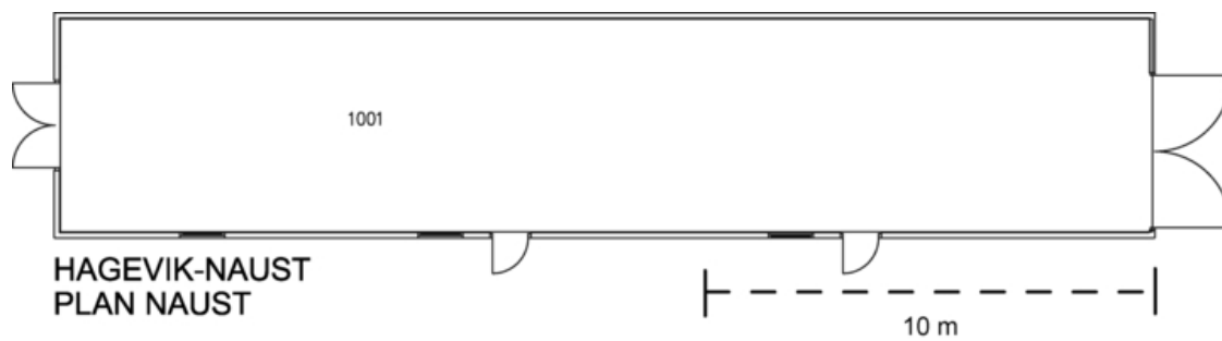
Plantegning 1. etasje.
