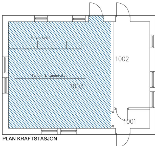
Plantegning av grunnplan.
