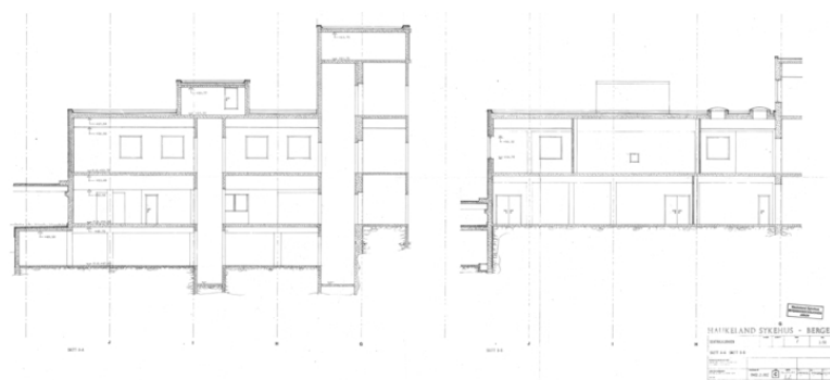
Snittegning A-A og B-B.
