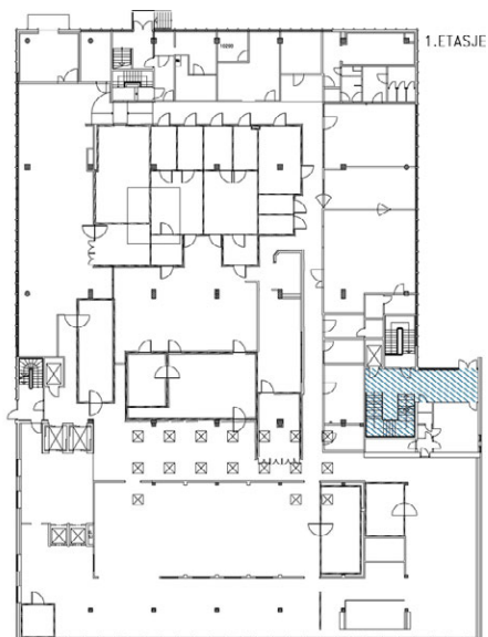
Plantegning 1. etasje.
