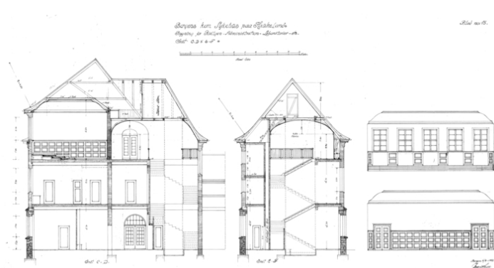
Snittegning etc. fra 1921.
