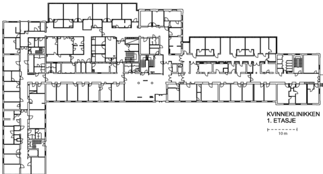
Plantegning 1. etasje.
