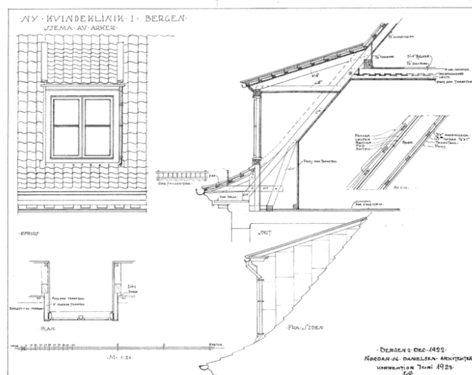
Tegning av arker mv.
