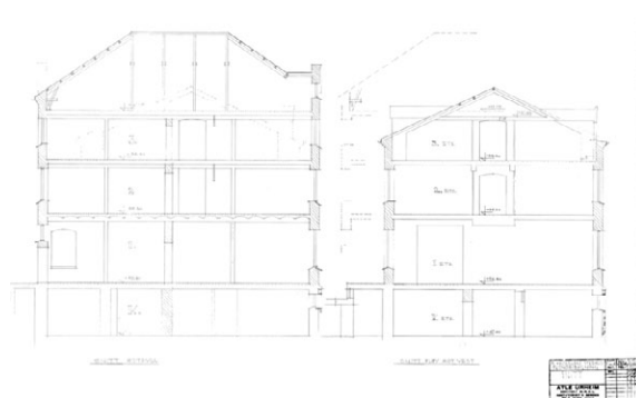
Snittegning midtbygg og mot vest.
