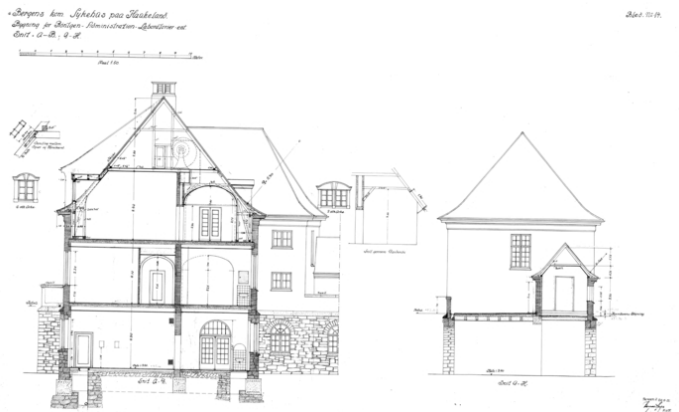
Snittegning etc. fra 1921.
