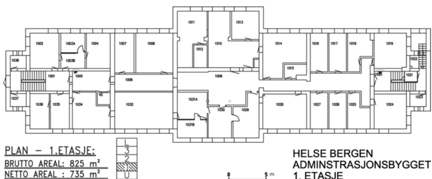
Plantegning, dagens situasjon.
