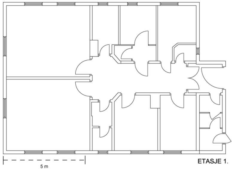
Plantegning 1. etasje.
