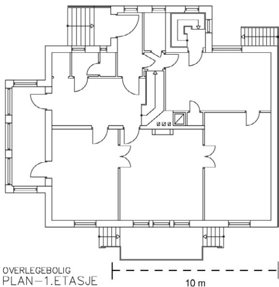
Plantegning 1. etasje.
