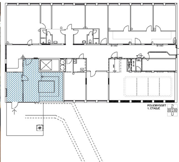
Plantegning 1. etasje.
