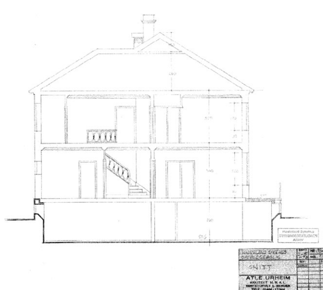
Snittegning.
