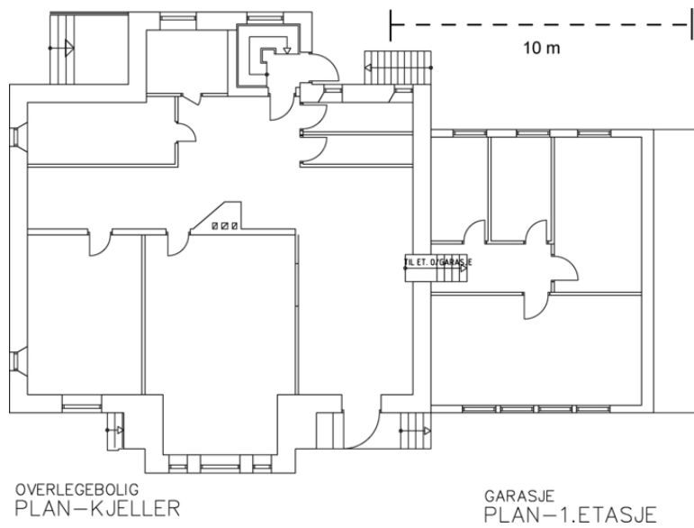
Plantegning underetasje.
