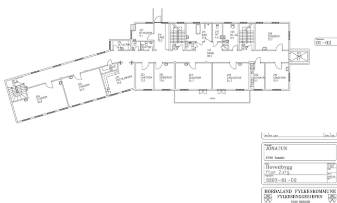
Plantegning hovedhus, 2. etasje.
