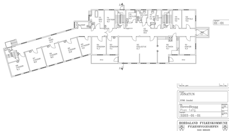
Plantegning hovedhuset, 1. etasje.
