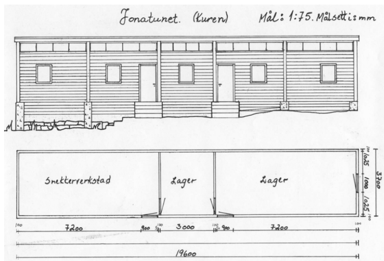
Fasade- og plantegning.
