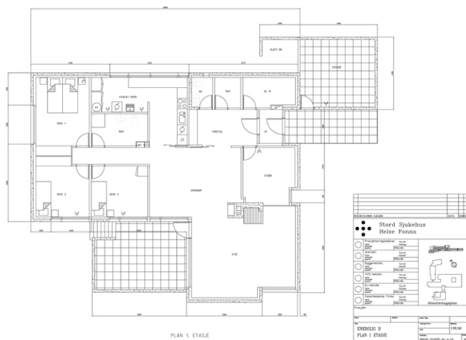
Plantegning bolig B.
