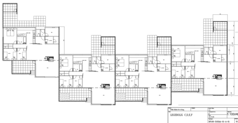
Plantegning boligene C-F.
