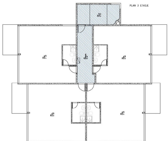
Plantegning 3. etasje.
