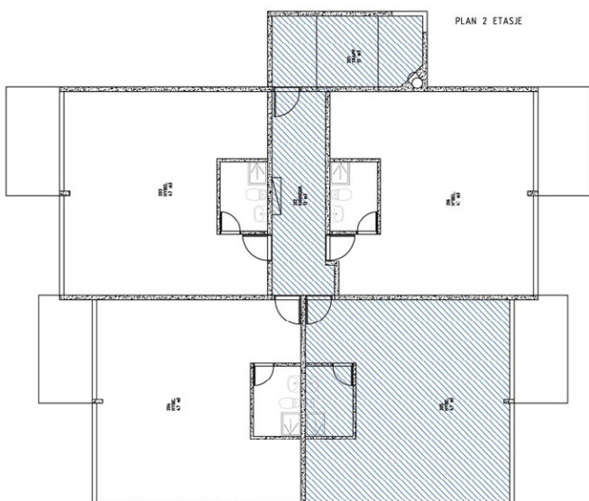
Plantegning 2. etasje.
