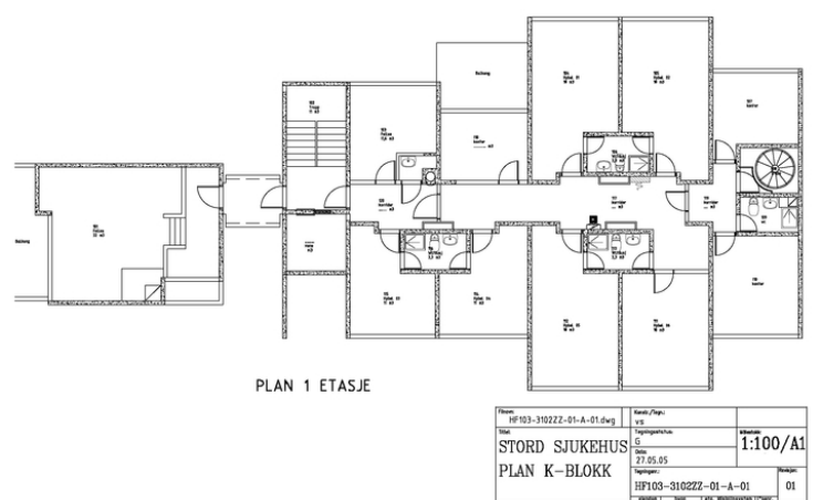
Plantegning 1. etasje blokk K.
