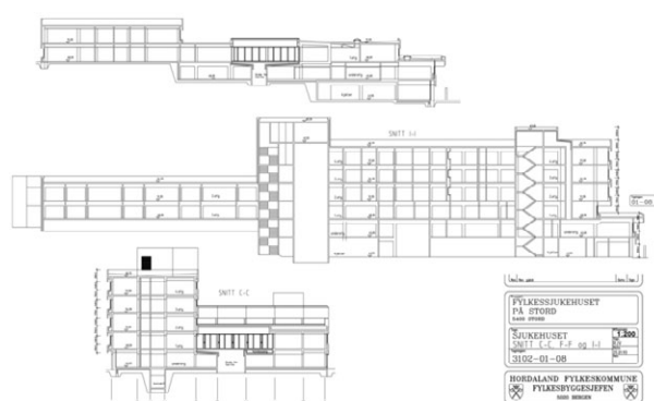
Snittegning hovedkompleks.
