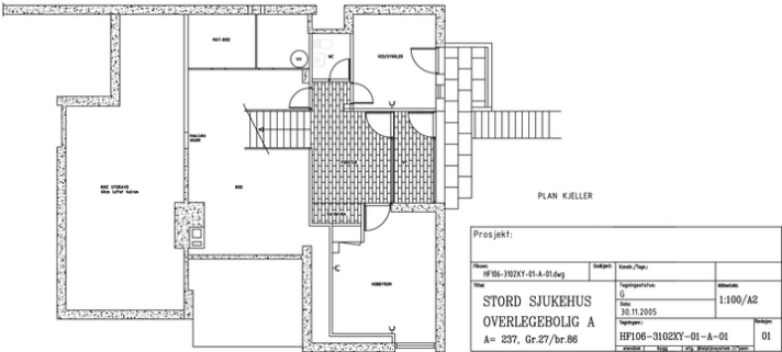
Plantegning kjeller.
