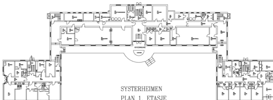
Plantegning 1. etasje.
