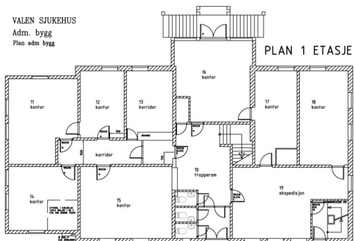
Plantegning 1. etasje.
