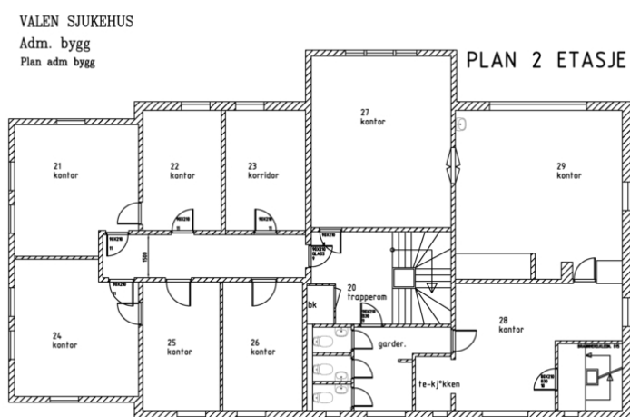
Plantegning 2. etasje.
