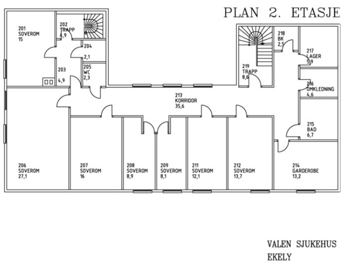
Plantegning 2. etasje.
